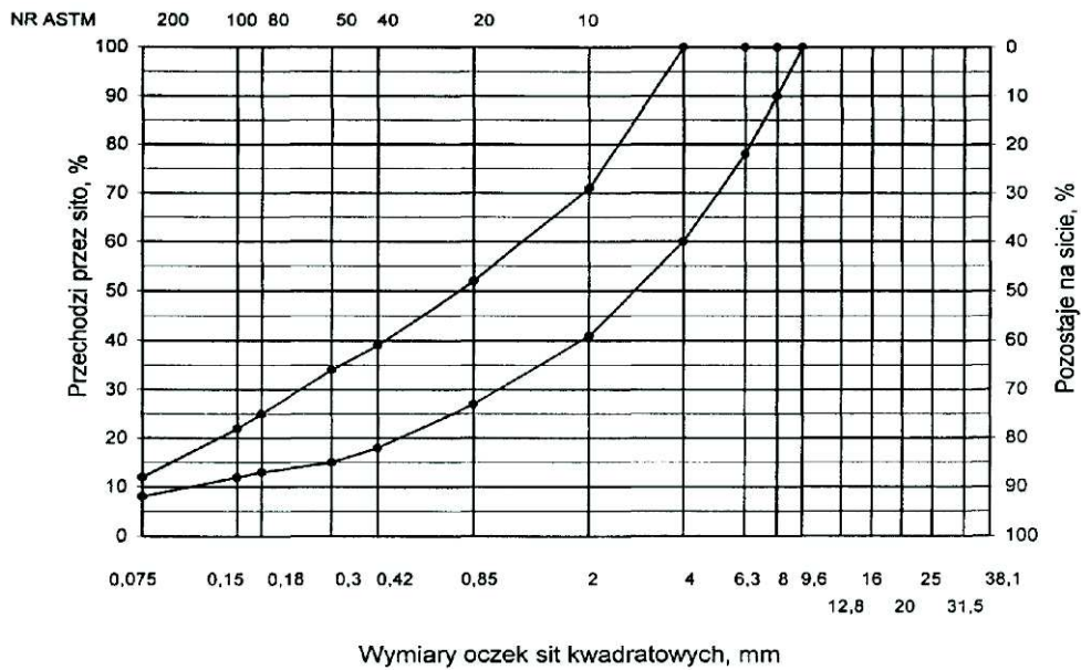
Rys. 3. Krzywe graniczne uziarnienia mieszanki mineralnej BA od 0 do 8mm, od 0 do 6,3 mm do warstwy ściernalnej nawierzchni drogi o obciążeniu ruchem nawierzchni drogi o obciążeniu ruchem KR1 lub KR2
