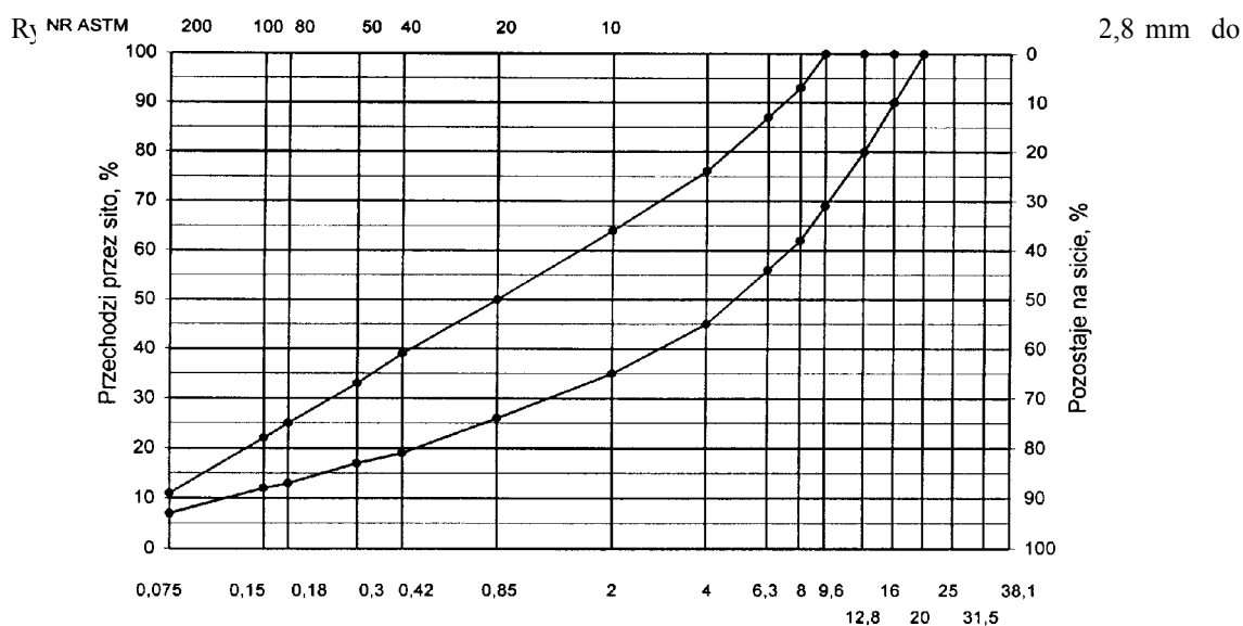
Rys. 1. Krzywe graniczne uziarnienia mieszanki mineralnej BA od 0 do 20 mm do warstwy ścieralnej nawierzchni drogi o obciążeniu ruchem dla KR1 lub KR2
