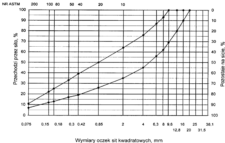
Rys. 2. Krzywe graniczne uziarnienia mieszanki mineralnej BA od 0 do 16mm, od 0 do 12,8 mm do warstwy ściernej nawierzchni drogi o obciążeniu ruchem KR1 lub KR2
