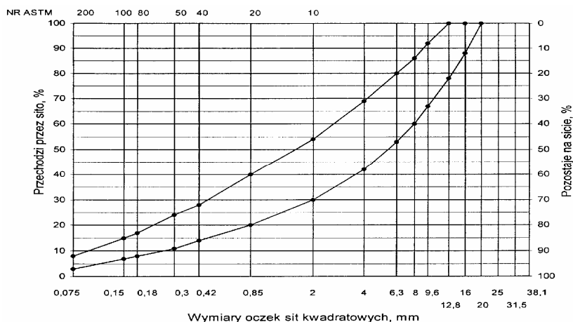
Rys. 9. Krzywe graniczne uziarnienia mieszanki mineralnej BA od 0 do 16 mm do warstwy wiążącej, wyrównawczej i wzmacniającej nawierzchni drogi o obciążeniu ruchem KR1 lub KR2
