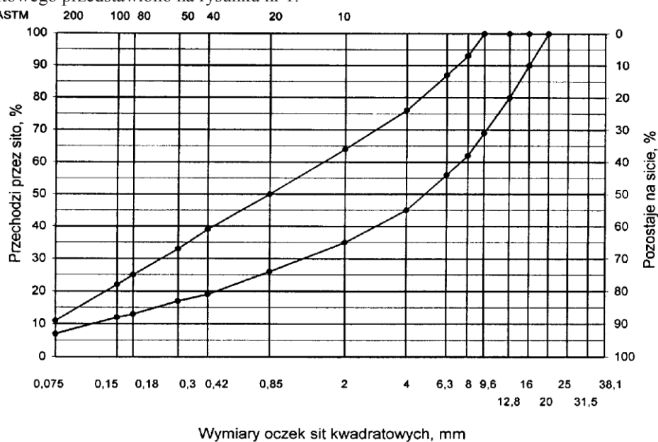
Rys. 1. Krzywe graniczne uziarnienia mieszanki mineralnej BA od 0 do 16mm, od 0 do 12,8 mm do warstwy ścieralnej nawierzchni
