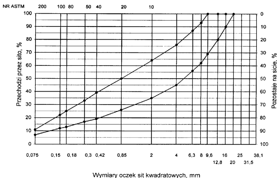
Rys. 1. Krzywe graniczne uziarnienia mieszanki mineralnej BA od 0 do 16mm, od 0 do 12,8 mm do warstwy ścieralnej nawierzchni
