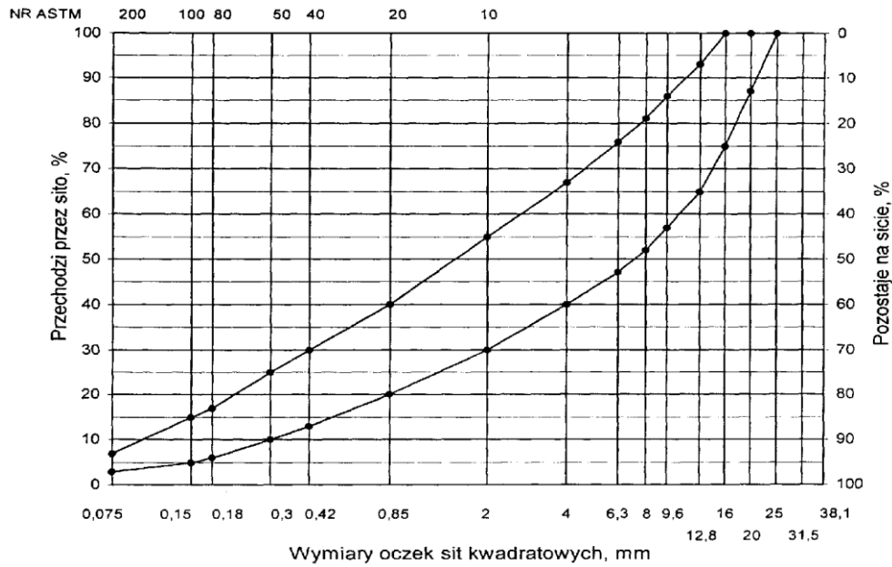
Rys. 2. Krzywe graniczne uziarnienia mieszanki mineralnej BA od 0 do 20 mm do warstwy wiążącej nawierzchni drogi o obciążeniu ruchem KR1 lub KR2
