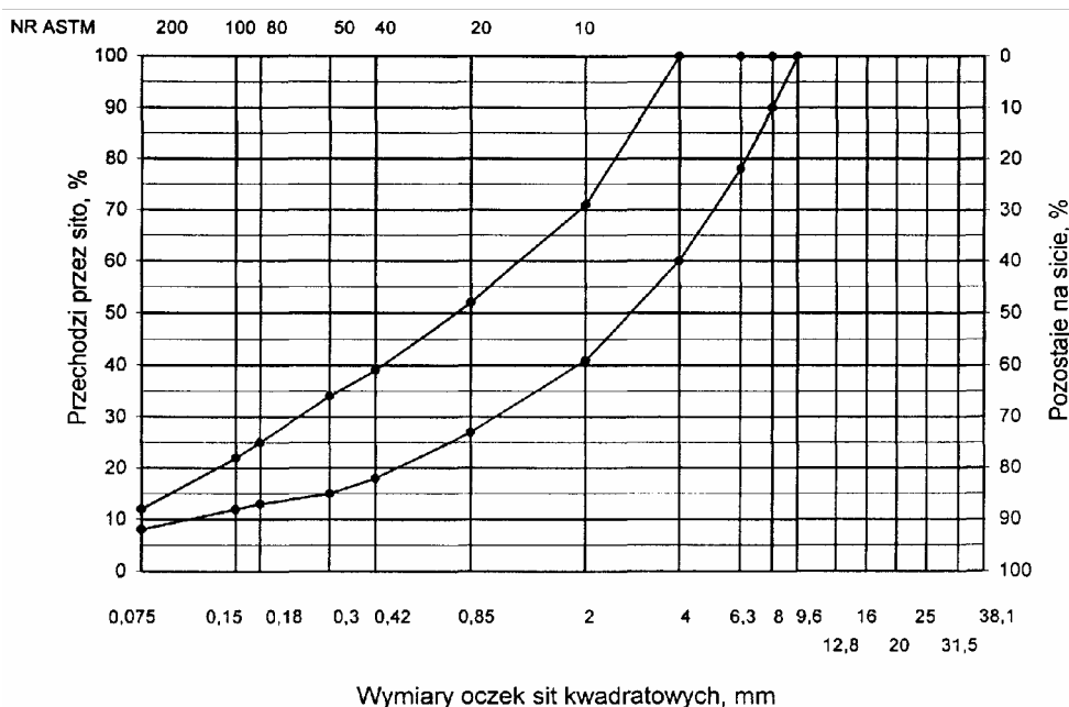
Rys. 1. Krzywe graniczne uziarnienia mieszanki mineralnej BA od 0 do 8mm, od 0 do 6,3 mm do warstwy ścieralnej nawierzchni ścieżki rowerowej
