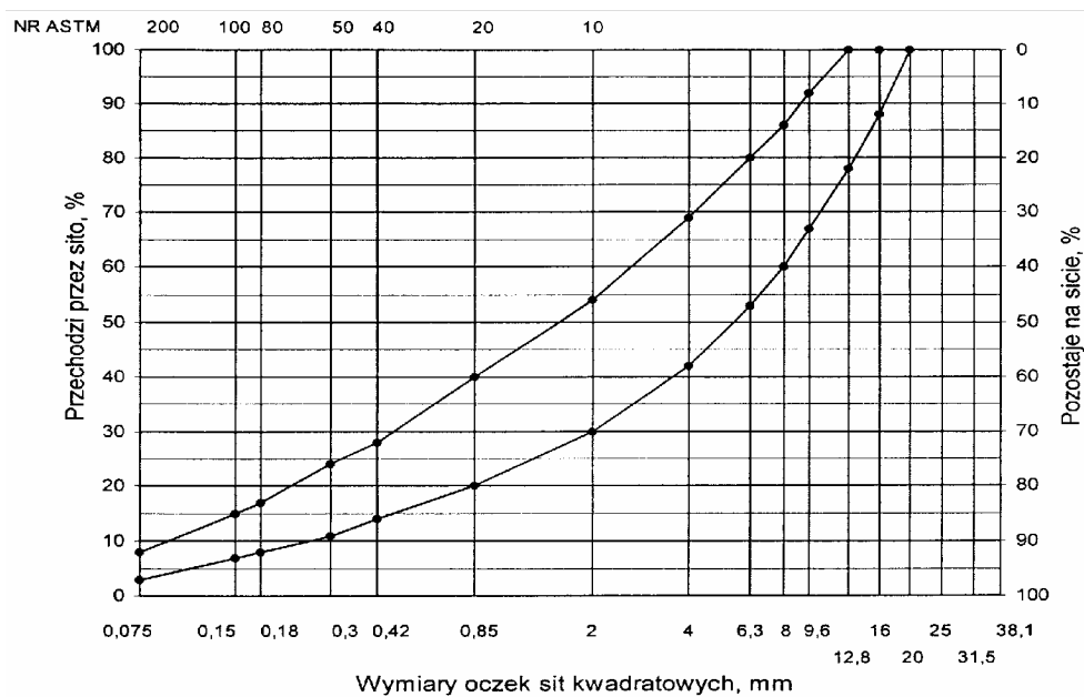
Rys. 2. Krzywe graniczne uziarnienia mieszanki mineralnej AC od 0 do 16 mm do warstwy wiążącej
